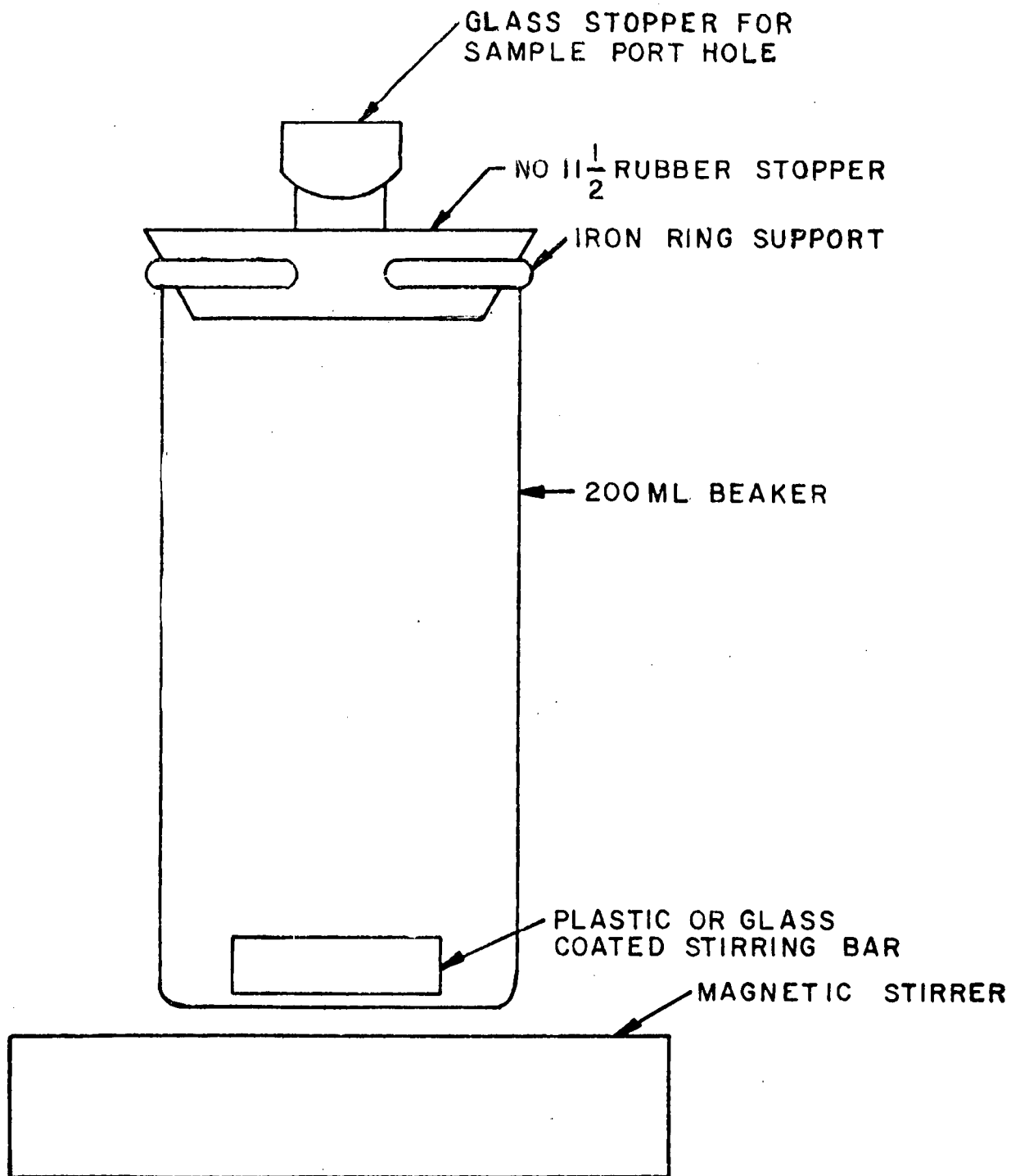
Fig 6. TITRATION ASSEMBLY
